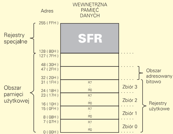
Rys. 3. Wewnętrzna pamięć danych w mikrokontrolerze 8051.
